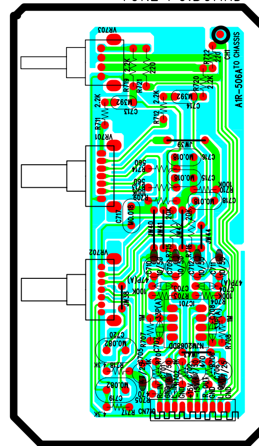
TONE PC.BOARD
